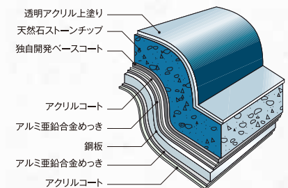
断面構成図
